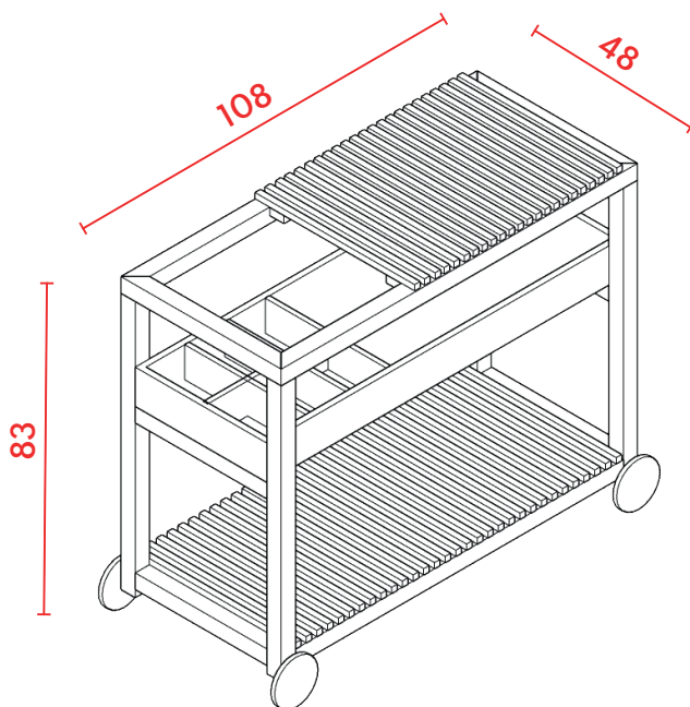
PERSPECTIVA
