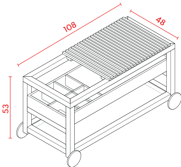
PERSPECTIVA
