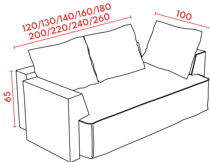
PERSPECTIVA
