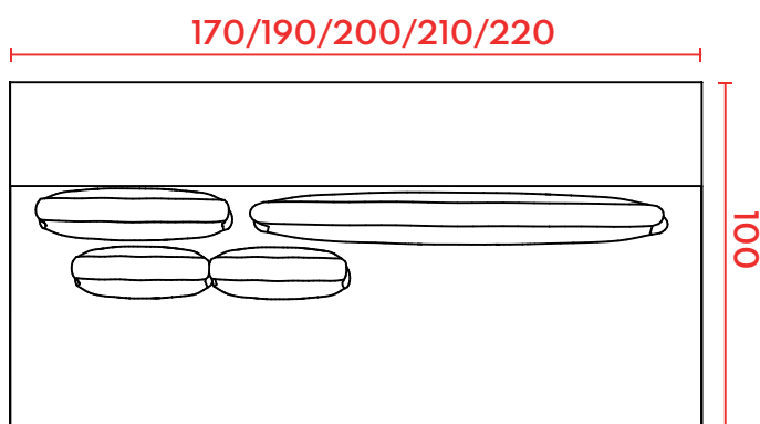
VISTA SUPERIOR
