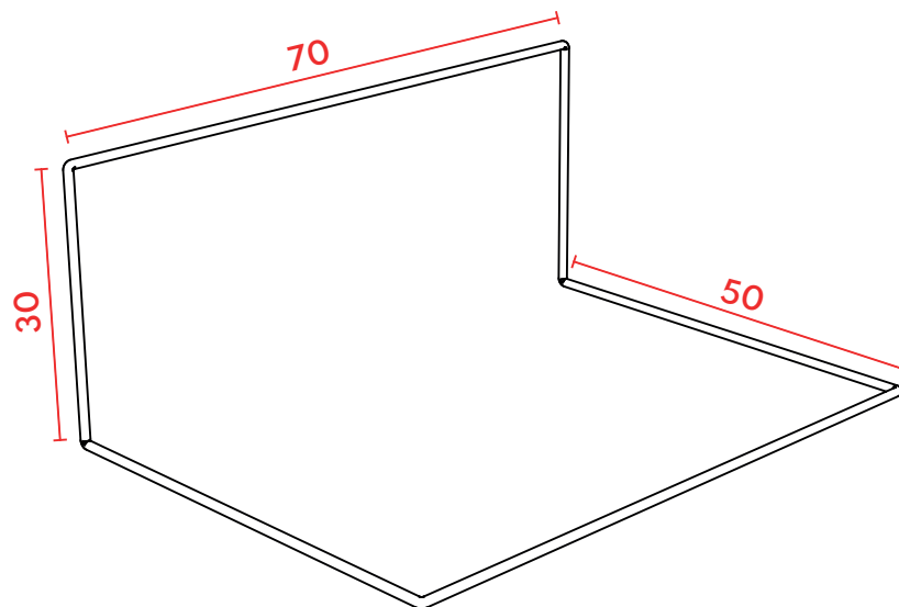
PERSPECTIVA
