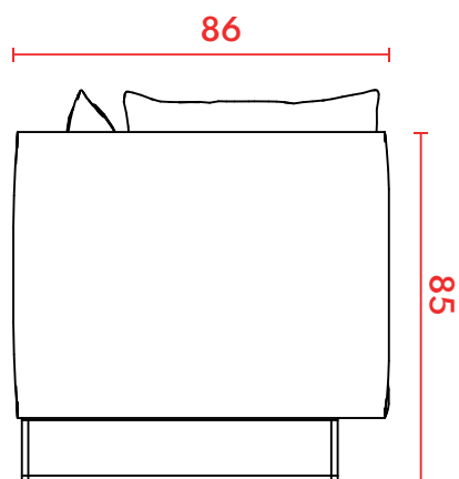
VISTA LATERAL ESQUERDA
