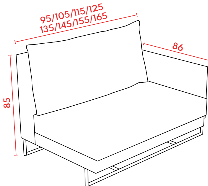
PERSPECTIVA
