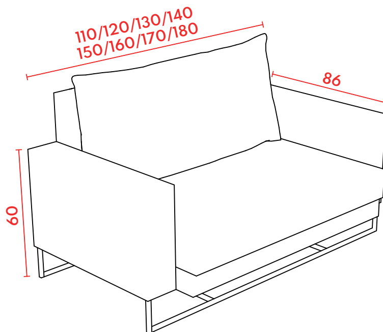
PERSPECTIVA
