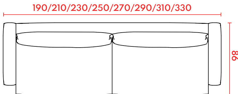
VISTA SUPERIOR
