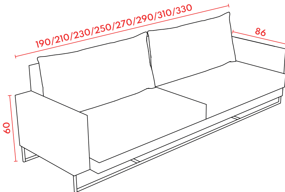
PERSPECTIVA
