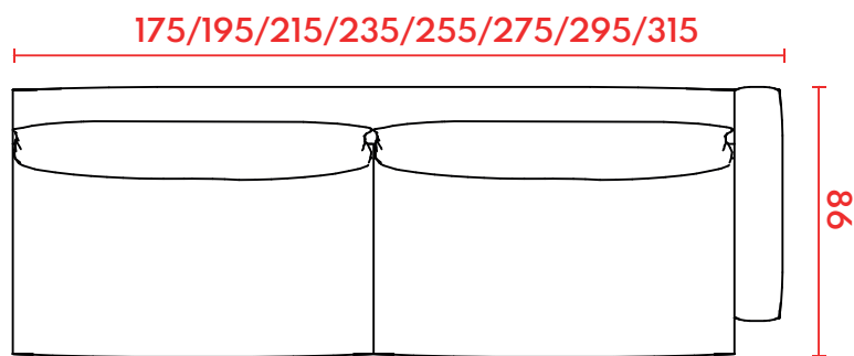
VISTA SUPERIOR
