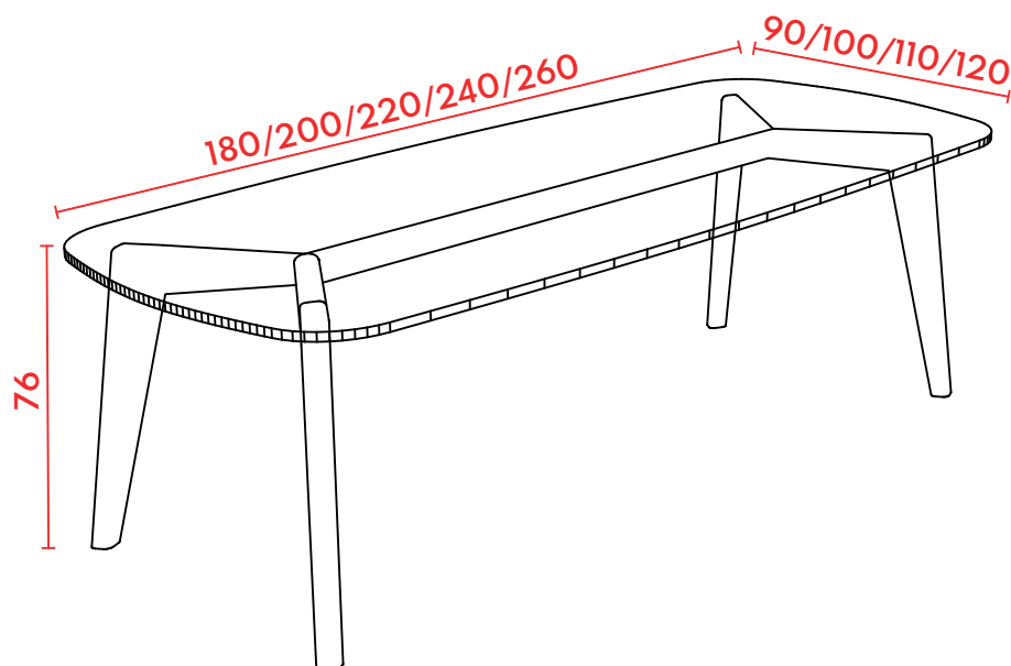
PERSPECTIVA
