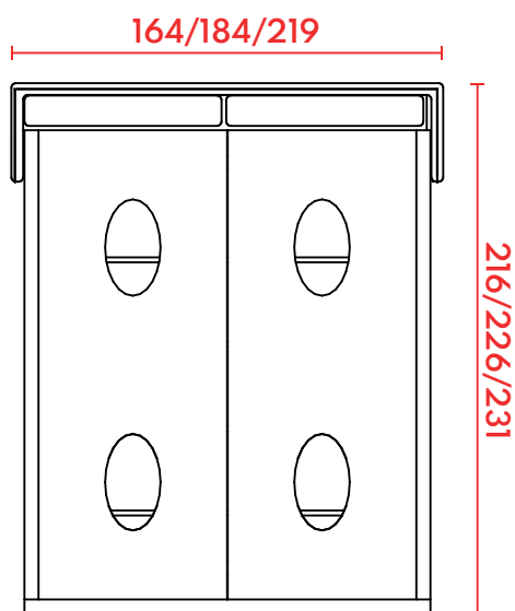
VISTA SUPERIOR
