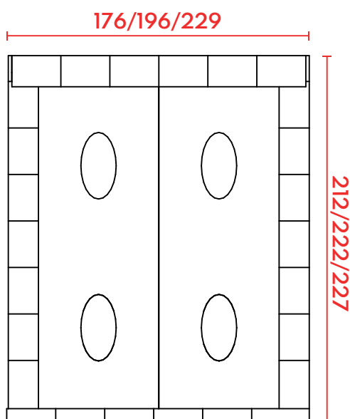
VISTA SUPERIOR
