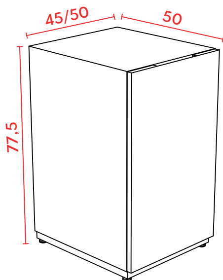
PERSPECTIVA
