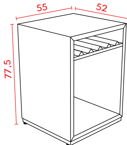
PERSPECTIVA
