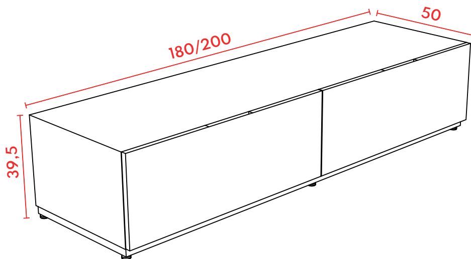
PERSPECTIVA
