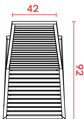
VISTA SUPERIOR
