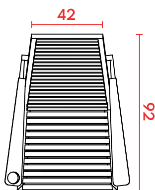
VISTA SUPERIOR
