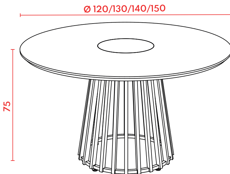
PERSPECTIVA
