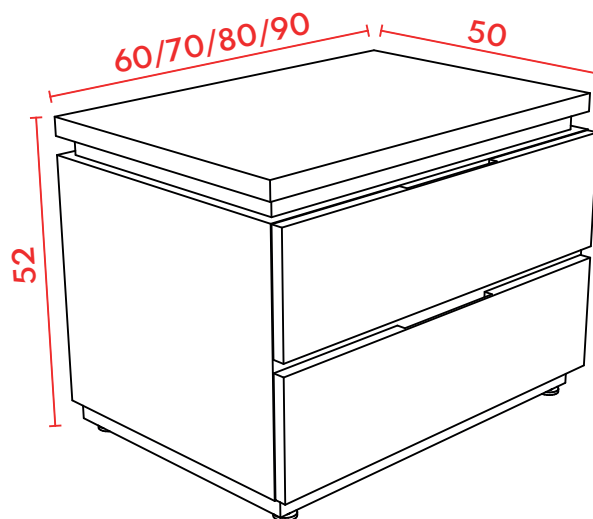
PERSPECTIVA
