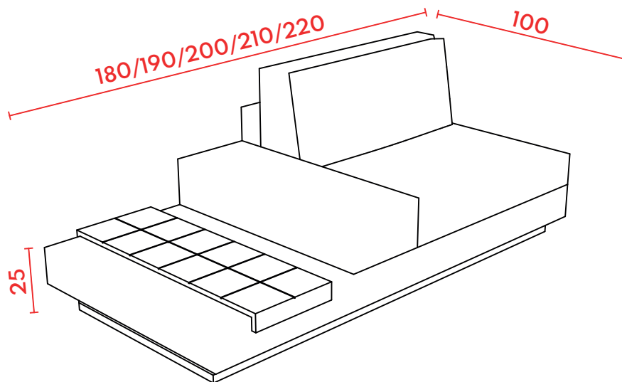
PERSPECTIVA
