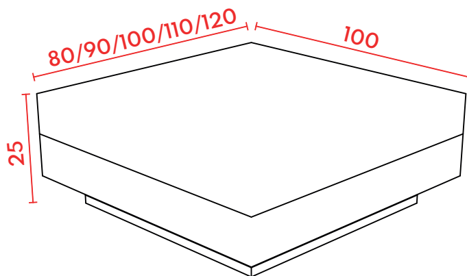
PERSPECTIVA
