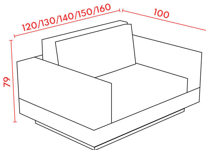
PERSPECTIVA
