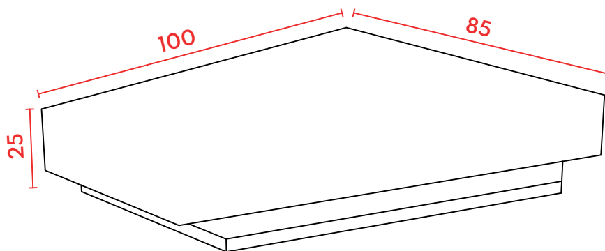
PERSPECTIVA
