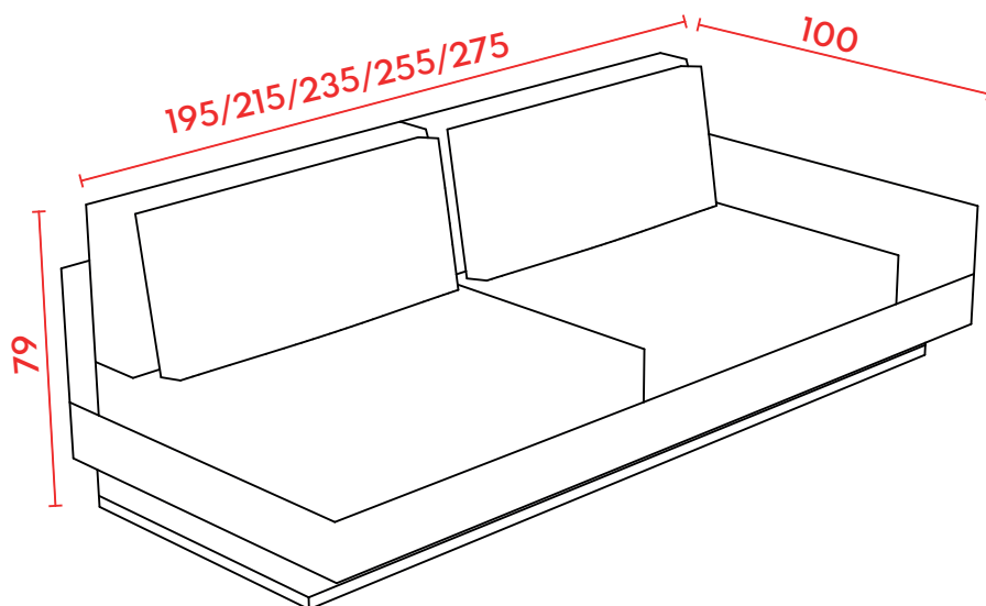
PERSPECTIVA
