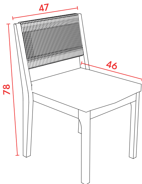
PERSPECTIVA
