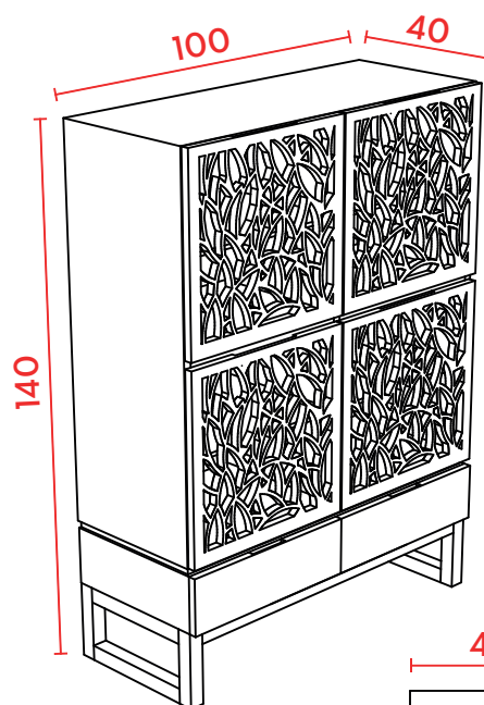
PERSPECTIVA
