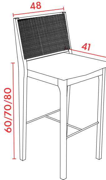
PERSPECTIVA
