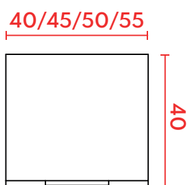
VISTA SUPERIOR
