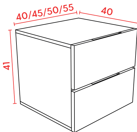
PERSPECTIVA
