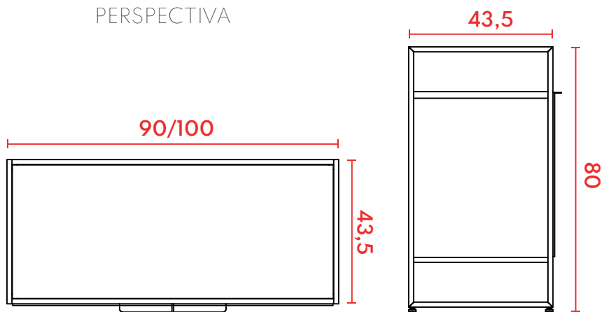
VISTA SUPERIOR
