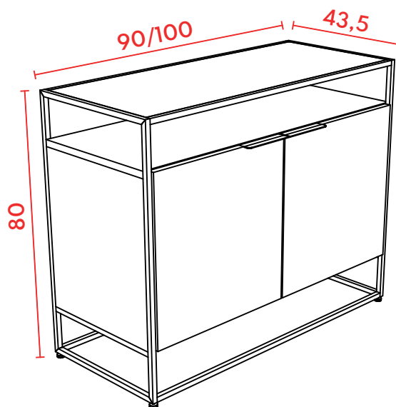
PERSPECTIVA
