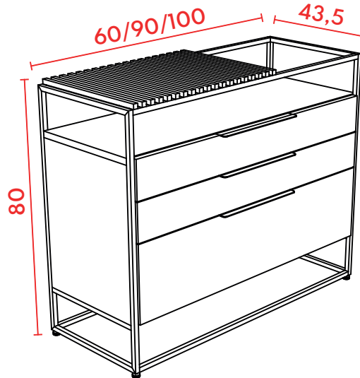
PERSPECTIVA
