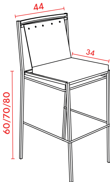
PERSPECTIVA
