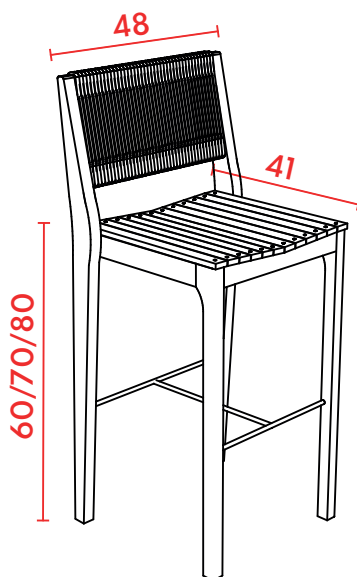
PERSPECTIVA
