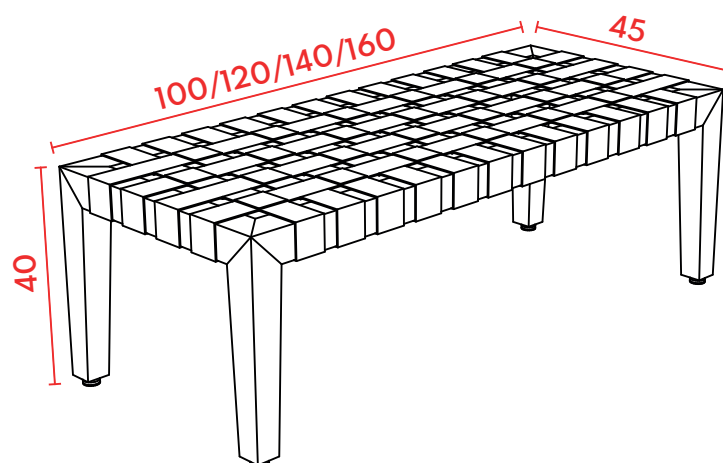
PERSPECTIVA
