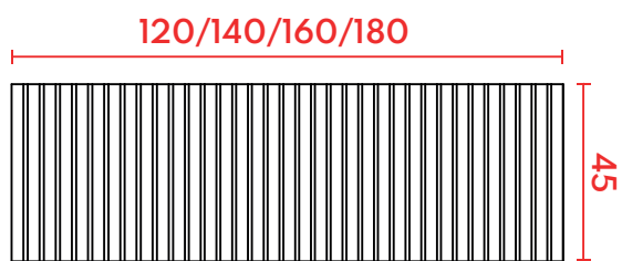
VISTA SUPERIOR
