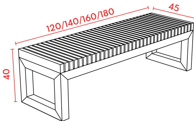
PERSPECTIVA
