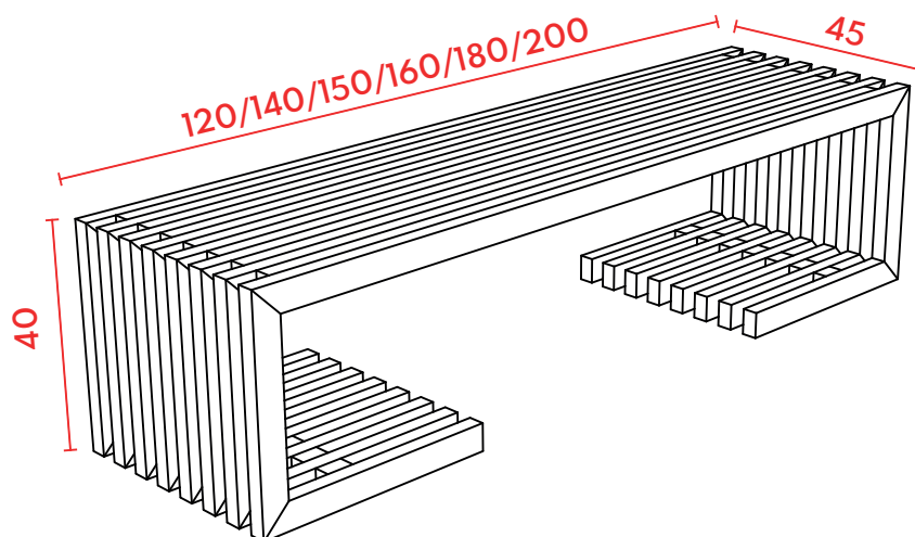
PERSPECTIVA
