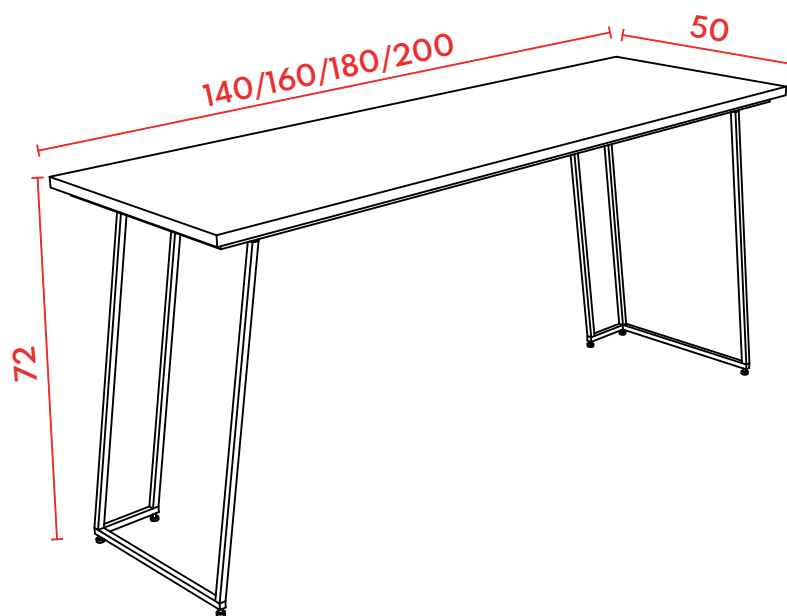
PERSPECTIVA
