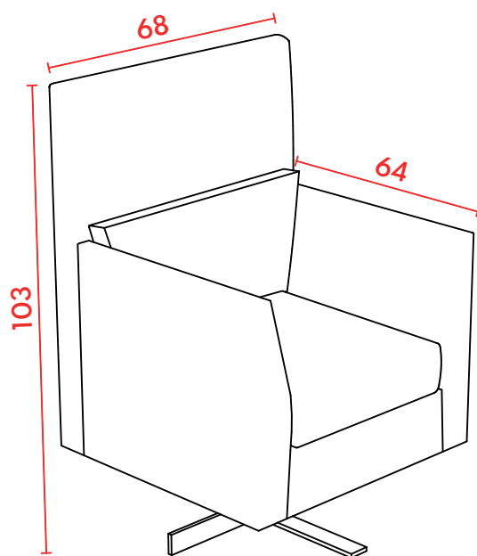
PERSPECTIVA
