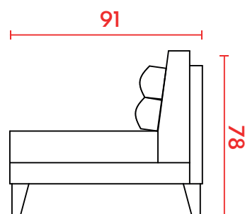
VISTA LATERAL DIREITA
