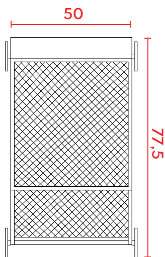
VISTA SUPERIOR
